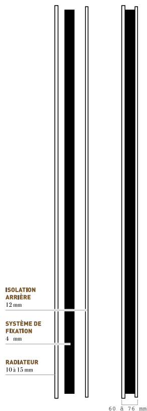
principe d'assemblage ultra-plat & isolant vue de profil en mm
